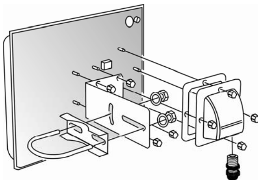
Abbildung 1-5. Befestigung der Abdeckplatte am TR-WMX-3.5
