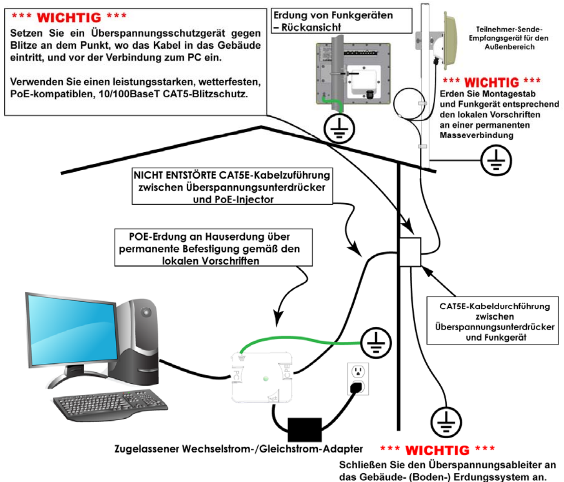
Abbildung 1-6. Beispiel für eine TR-WMX-3.5-Installation
