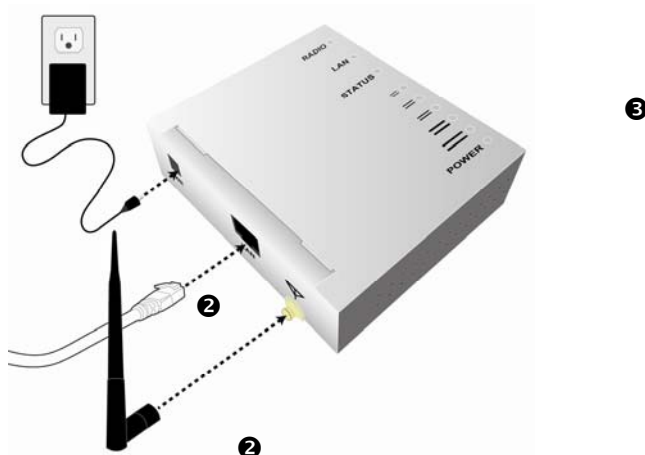
Abbildung 1-7. Installation der Innenbereichskomponente
